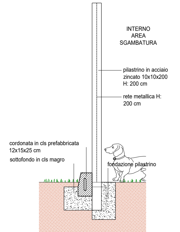
PARTICOLARE RECINZIONE PERIMETRALE
